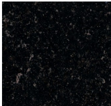
Neptunite
